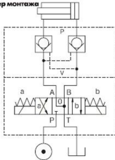
Пример монтажа
